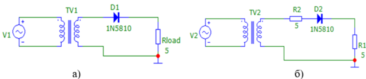
Малюнок 2 – Схема дослідження однонапівперіодної схеми (а) та модифікован схема для побудови характеристики навантаження (б)
