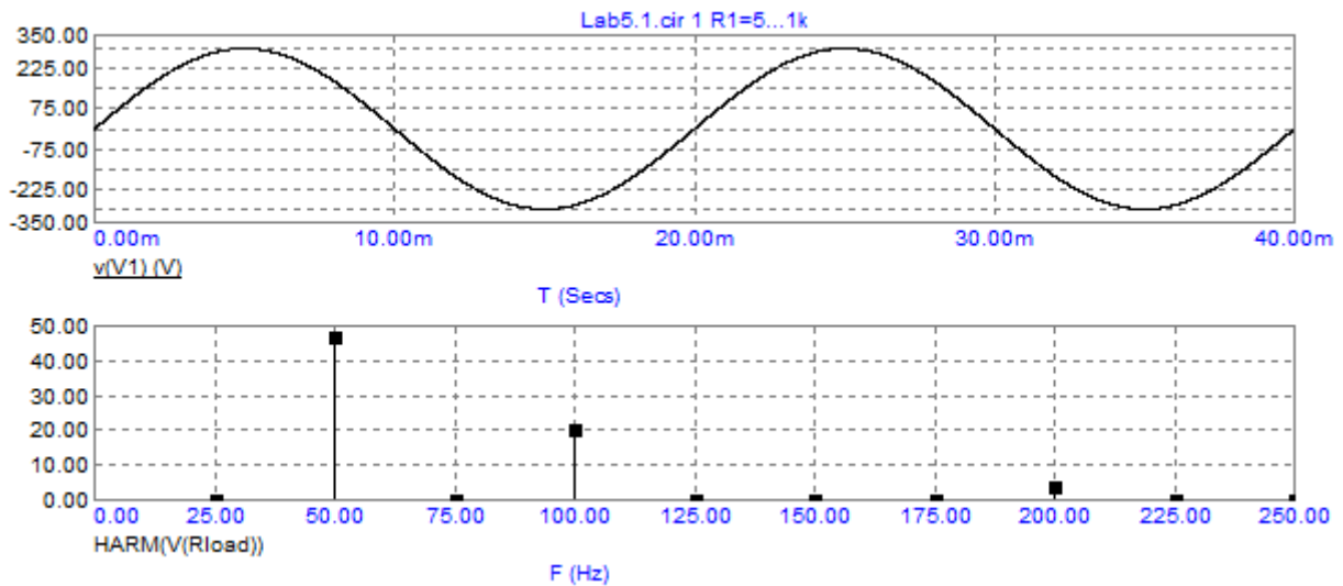
Малюнок 4 – Графічні залежності напруги вторинної обмотки та ряд гармонік
