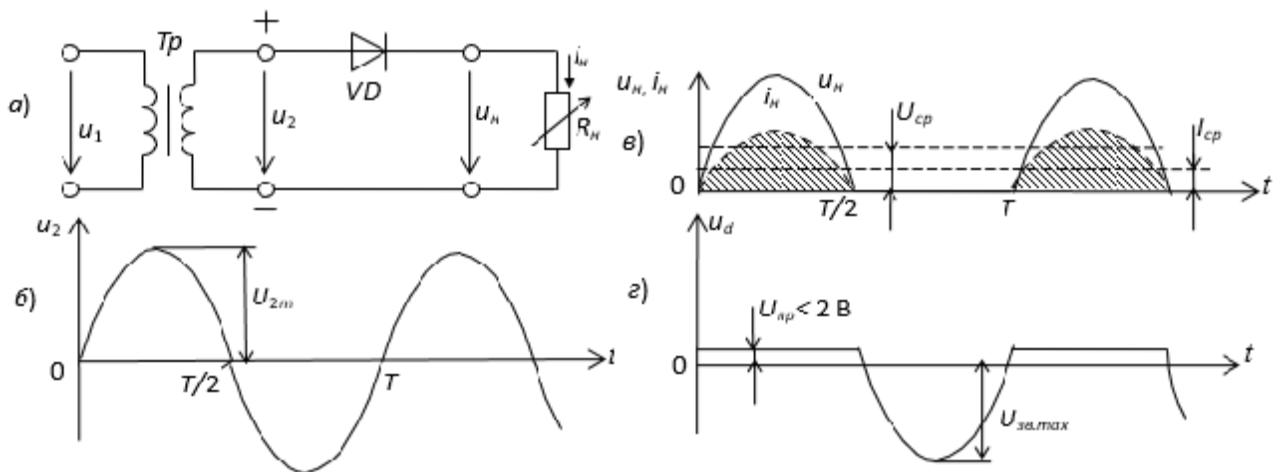
Малюнок 1 – Однонапівперіодна схема випрямлення (а), часова діаграма вторинної обмотки трансформатору (б), часові діаграми напруги і струму на навантаженні (в), часова діаграма напруги на вентилі (г)
