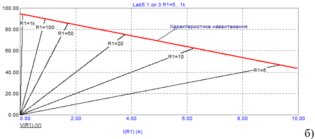
Малюнок 6 – Вікно налаштування та характеристика навантаження
