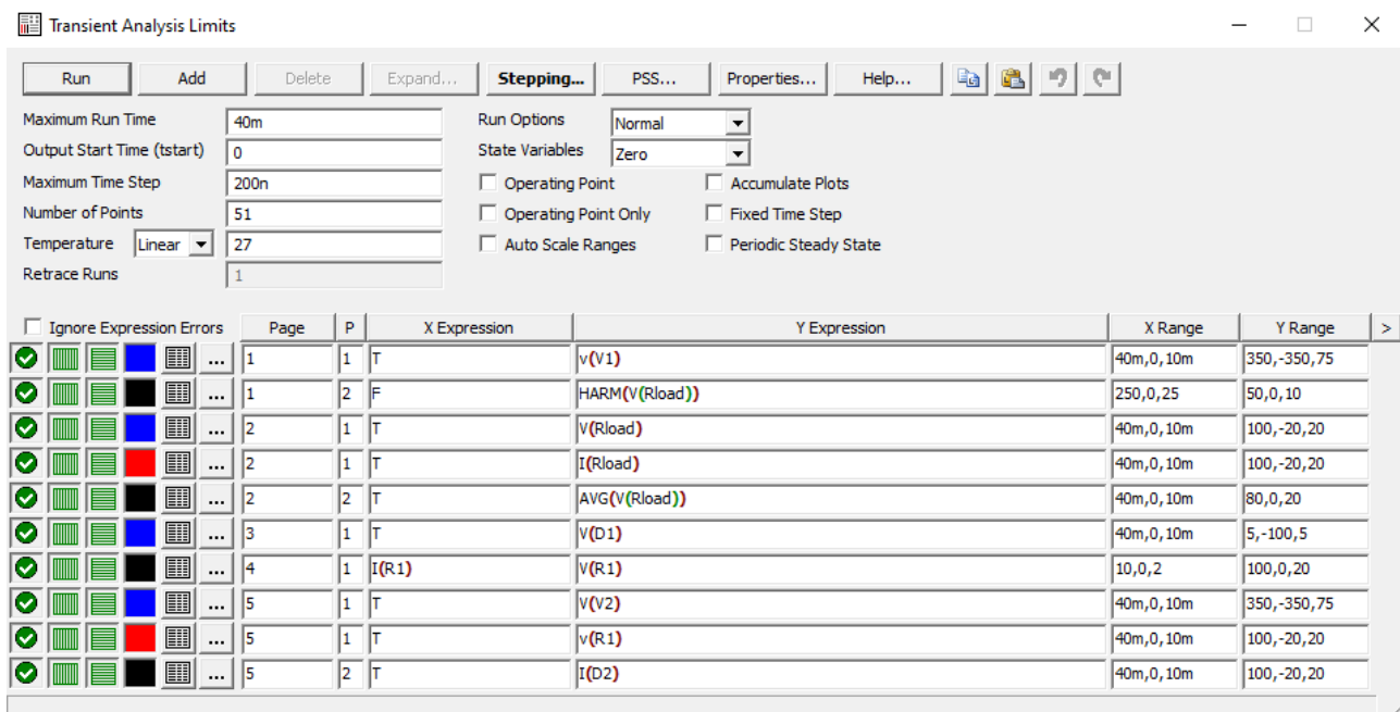
Малюнок 3 – Вікно налаштувань Transient Analysis
