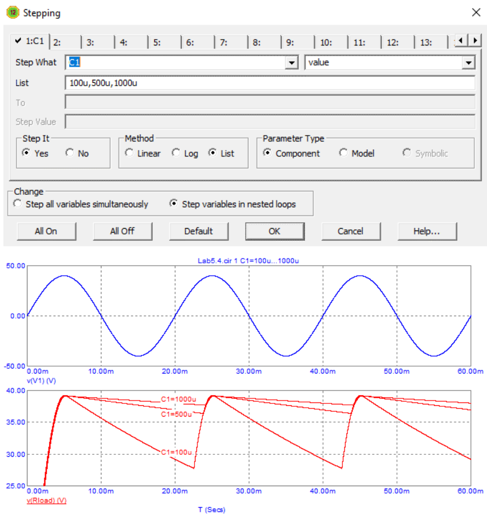
Рисунок 8 – Вікно налаштувань та графічні залежності впливу ємності згладжуючого фільтру
